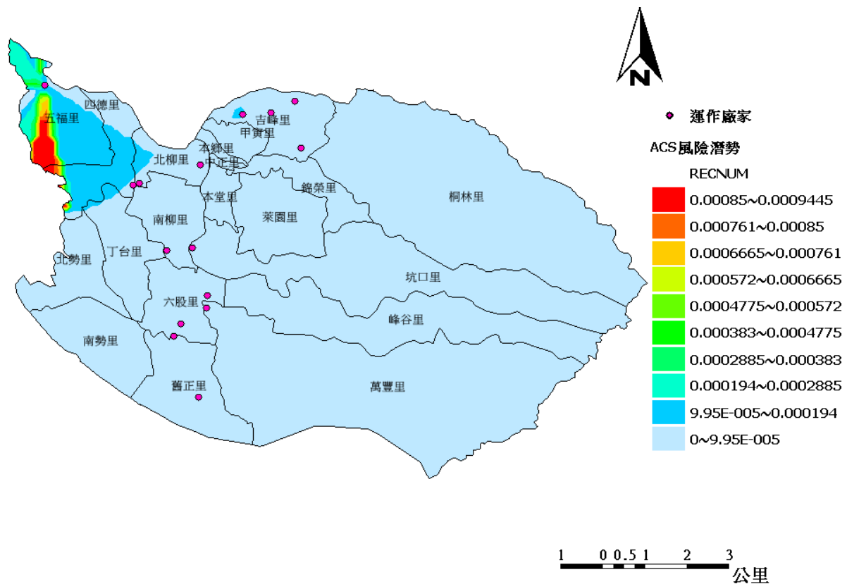
圖 1-3-35 臺中市霧峰區一般洩漏模擬情境(ACS)毒性及關注化學物質災害潛勢圖
