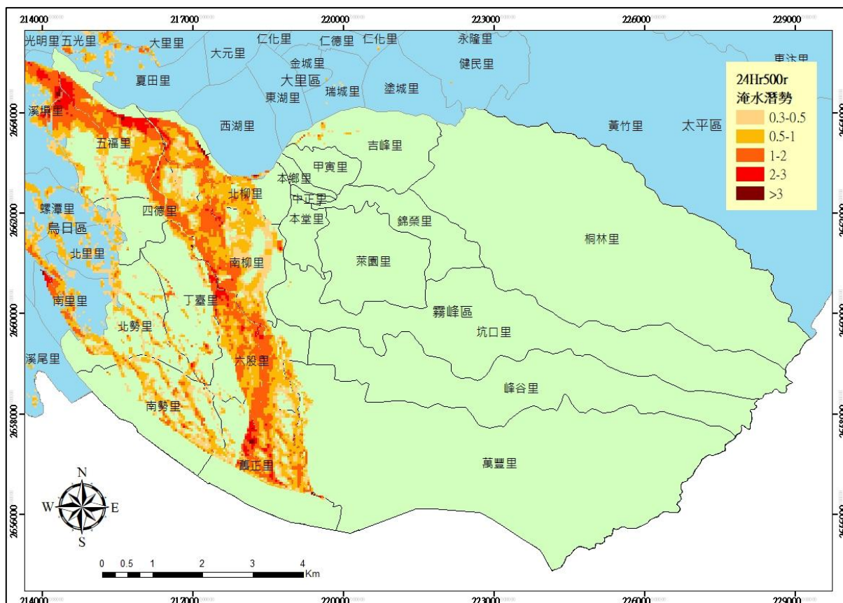
圖 1-3-25 霧峰區 24 小時累積 500 毫米淹水潛勢圖
