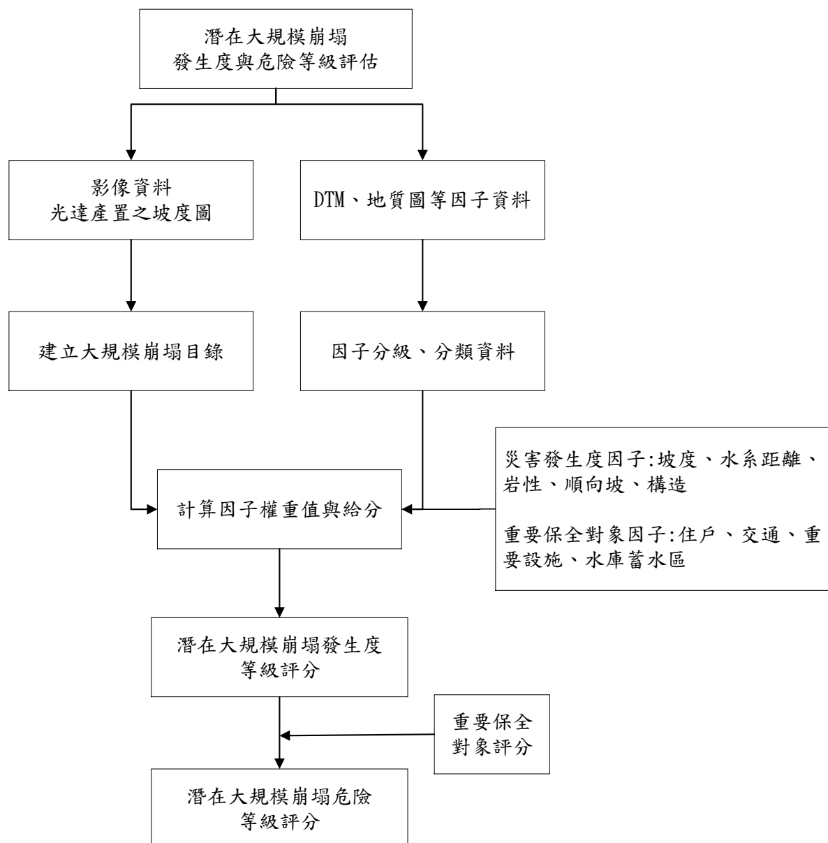
圖 1-3-29 大規模崩塌災害潛勢危害等級評估流程圖
