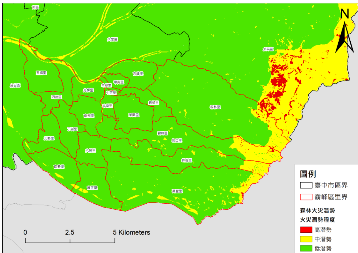
圖 1-3-38 臺中市霧峰區森林火災潛勢圖
