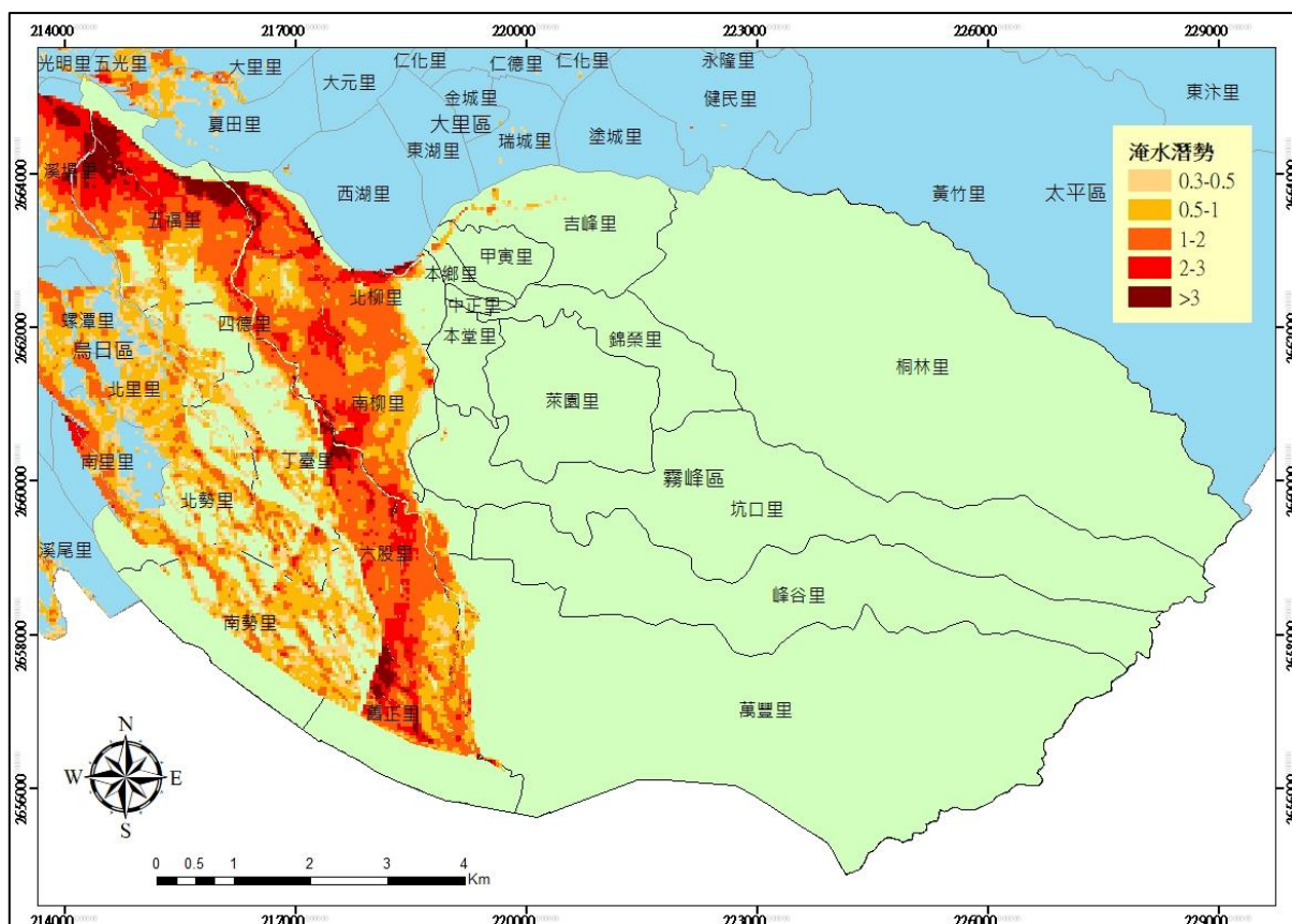
圖 1-3-26 霧峰區 24 小時累積 650 毫米淹水潛勢圖
