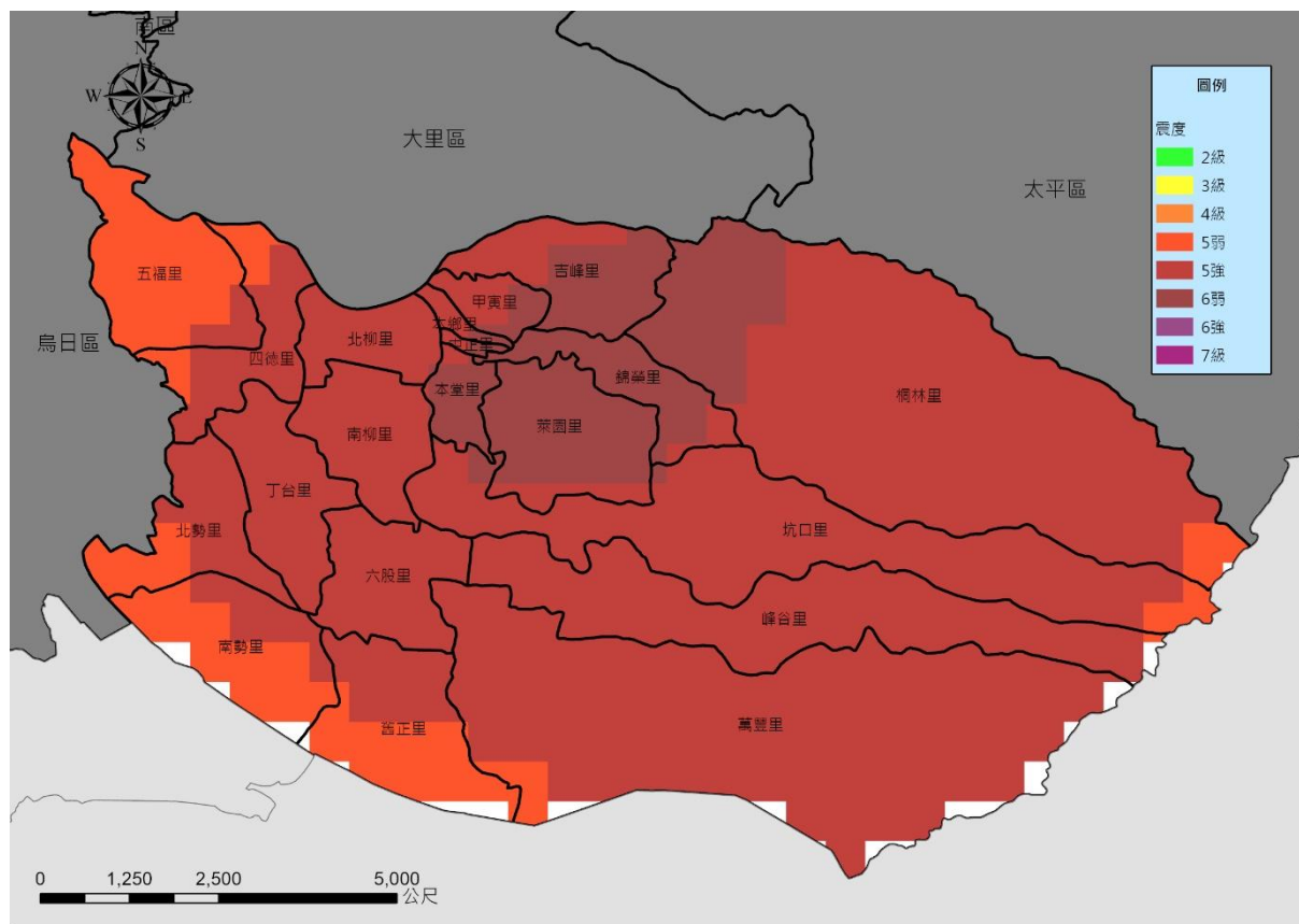
圖 1-3-6 本區車籠埔斷層最大地表加速度推估圖
