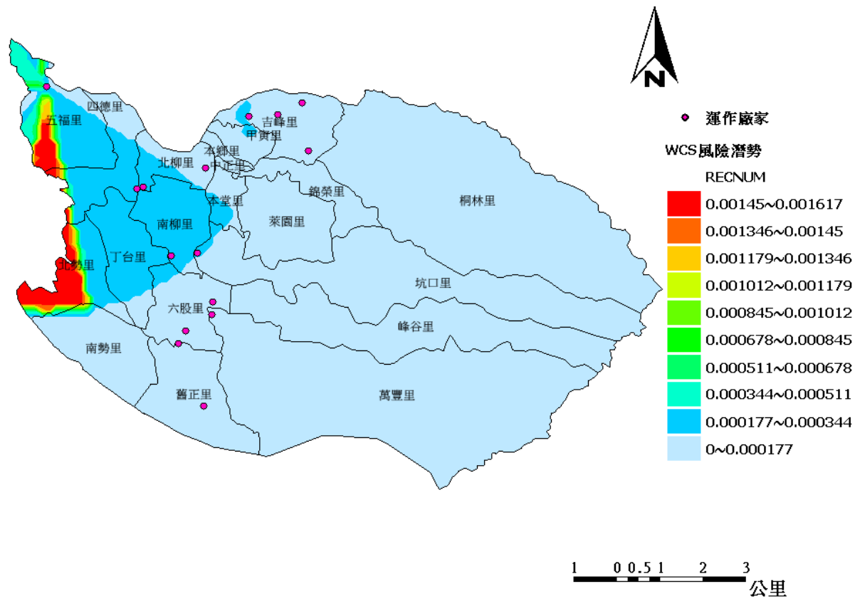
圖 1-3-34 臺中市霧峰區最嚴重洩漏模擬情境(WCS)毒性及關注化學物質災害潛勢圖
